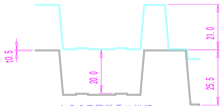
180度回転重ね詳細 (S=1/1)
