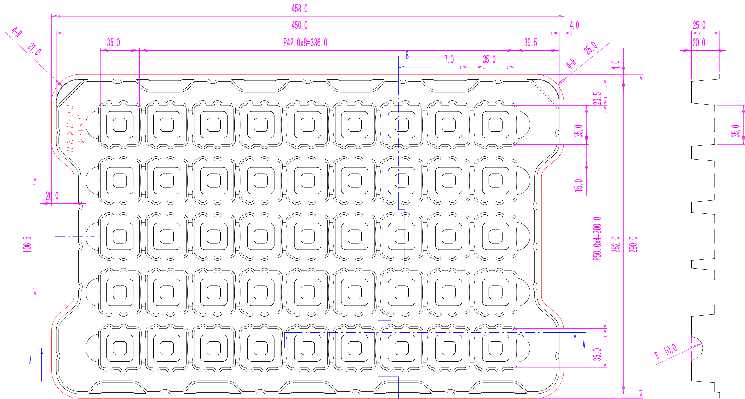
B - B 断面
