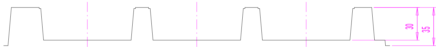
A - A 断面
