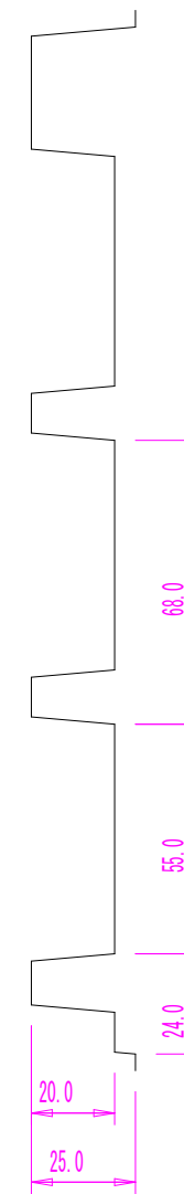
断面B-B
